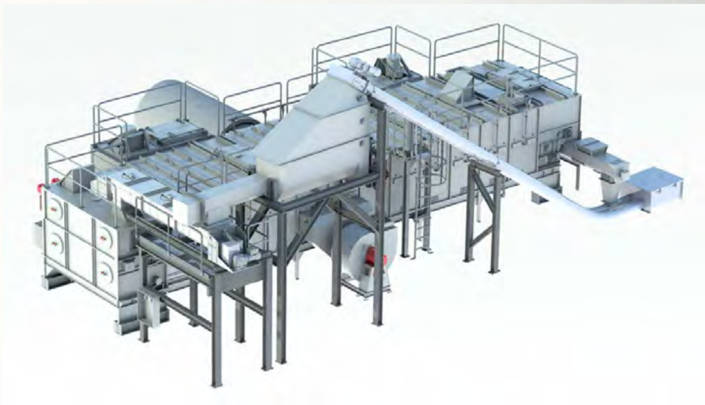
项目地：SC Ness Projekt Europe, 罗马尼亚 | 型号：BTLU 1/3000-12 | 安装年份：2024年 干燥物料：市政污泥 | 蒸发量：1.0吨/小时
